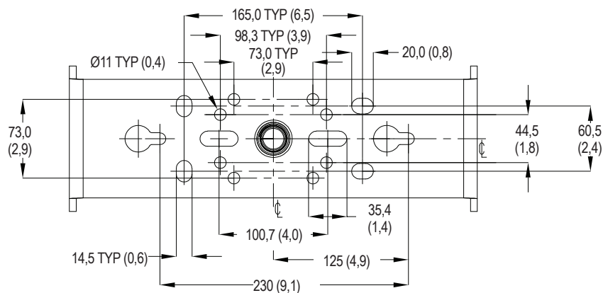
Vue de dessus du support
