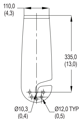
Vue latérale du support
