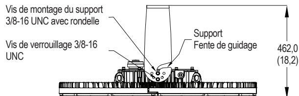
Vue de face du support
