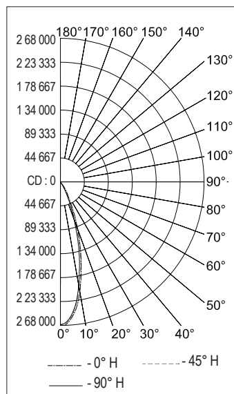
DISTRIBUTION DE TYPE POLAIRE (CANDELAS)
