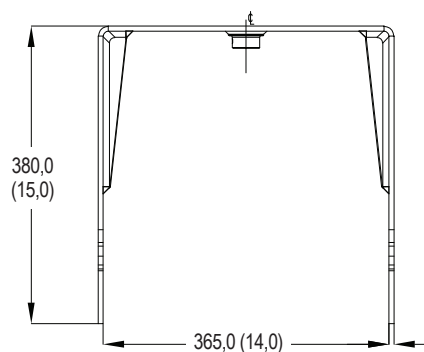
Vue de dessus du support
