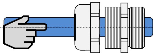
Toujours commencer le serrage à la main et finir à la clé Always begin the tightening by hand and finish with the key
