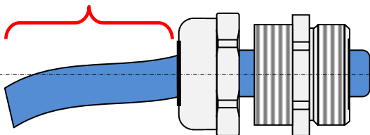
A éviter - Risque de forcer le filetage Avoid this- Risk of forcing the threading
